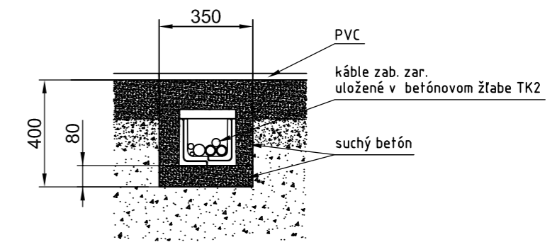
Uloženie káblov v DK ŽST Bošany
