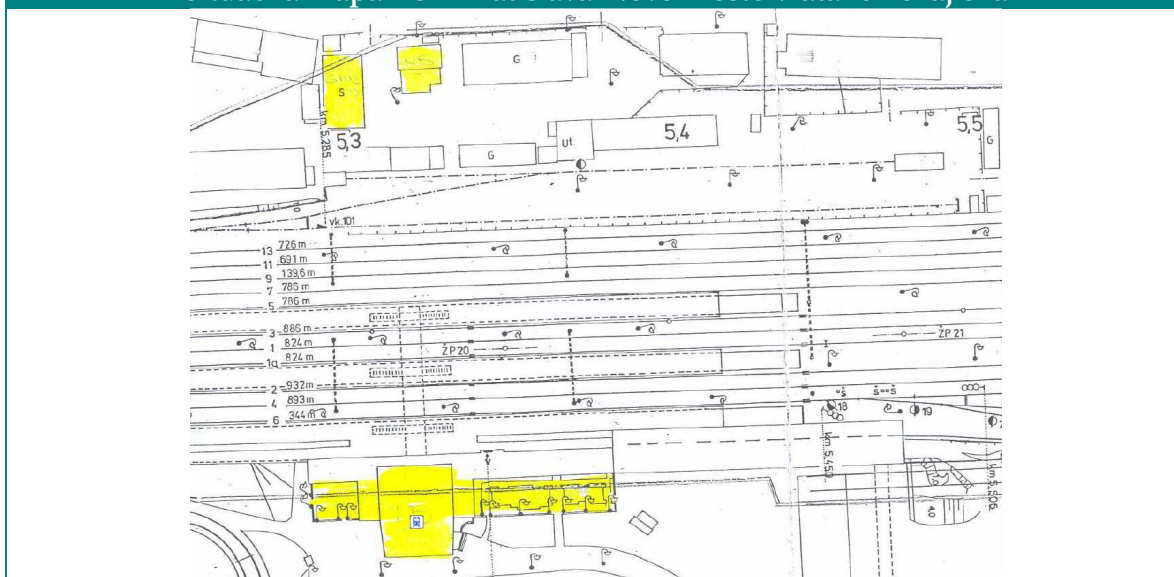
Situačná mapa ŽST Bratislava Nové Mesto vrátane koľajiska
